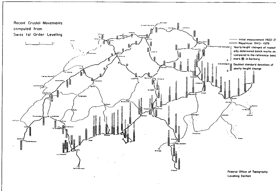
Fig. 2. - Velocità dei movimenti crostali verticali in Svizzera
